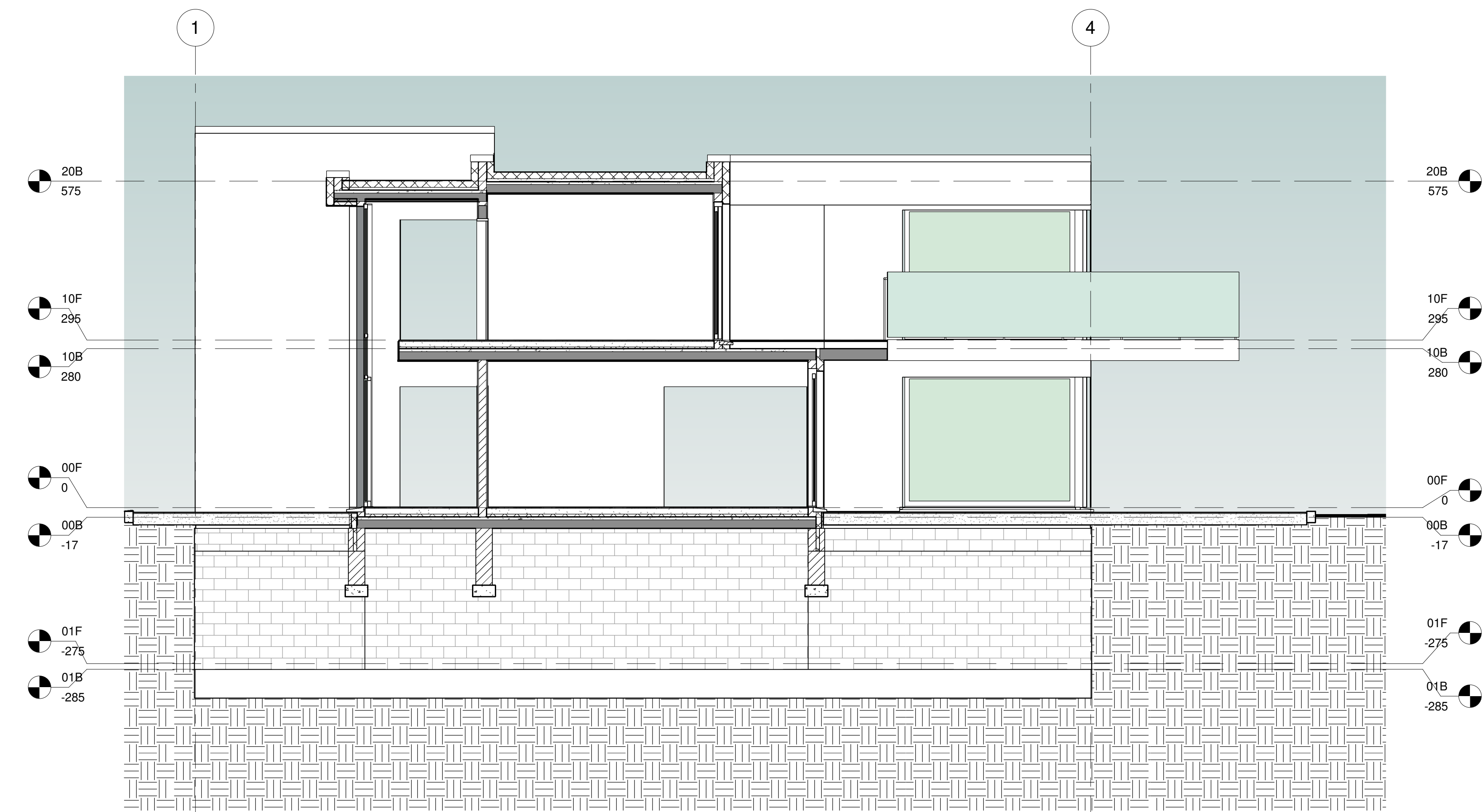
2 Coupe 2 1 : 50
