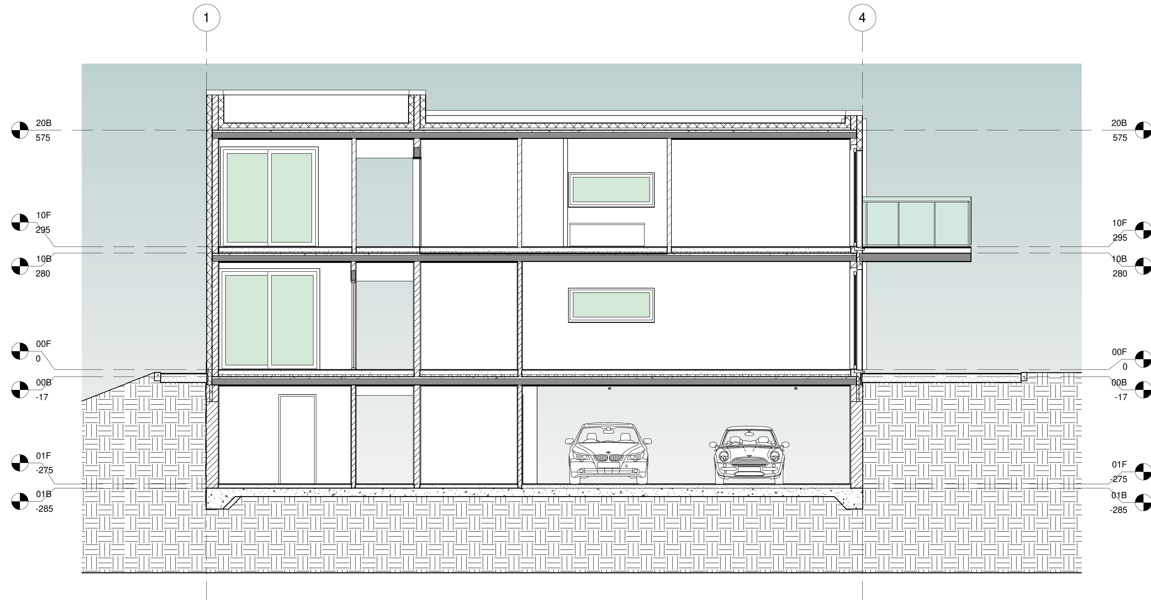
1 Coupe 1 1 : 50
