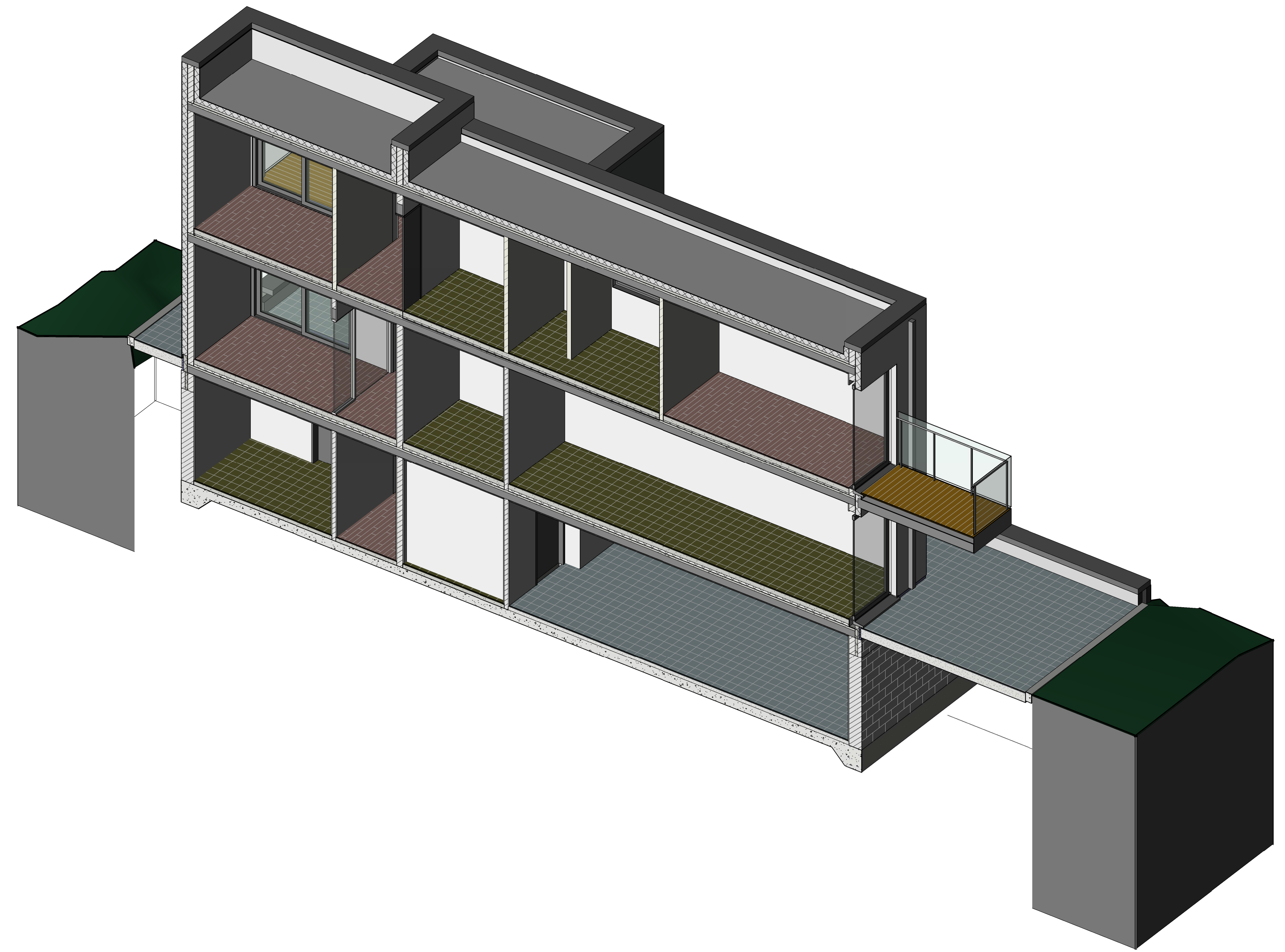
3 3D Coupe 1
