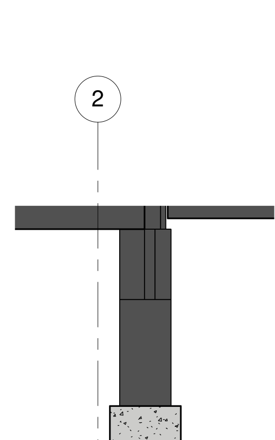
4 Coupe de détail 02 1 : 20
