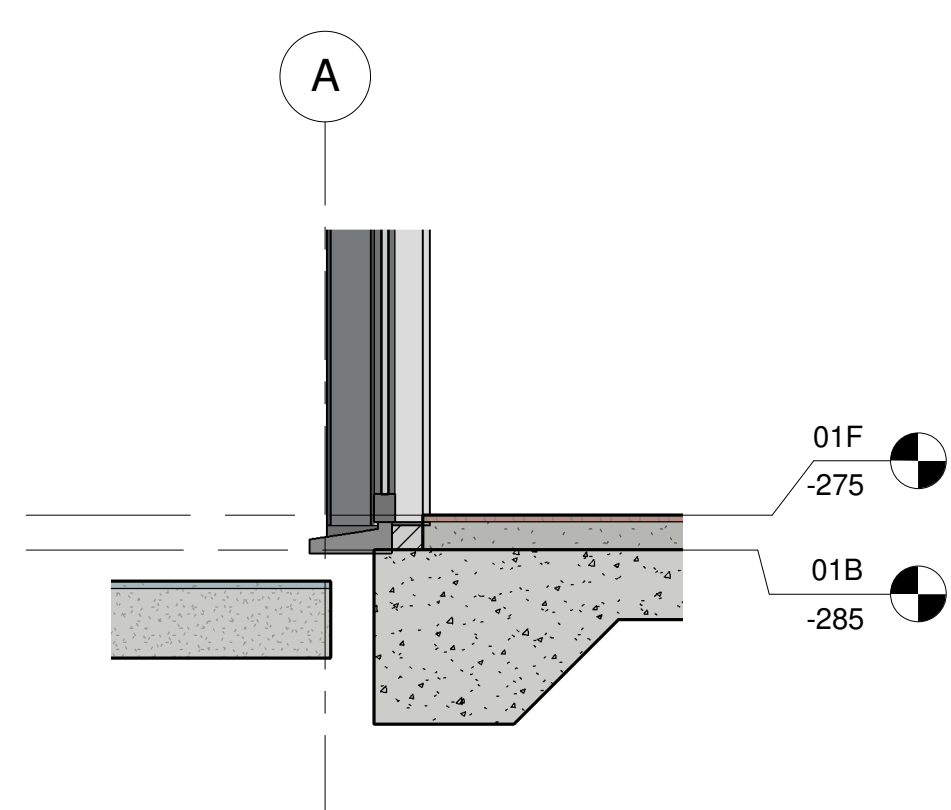
3 Coupe de détail 01 1 : 20
