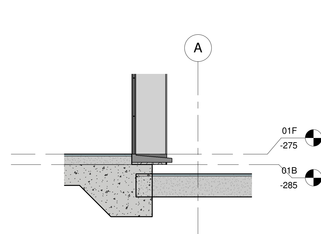
6 Coupe de détail 04 1 : 20
