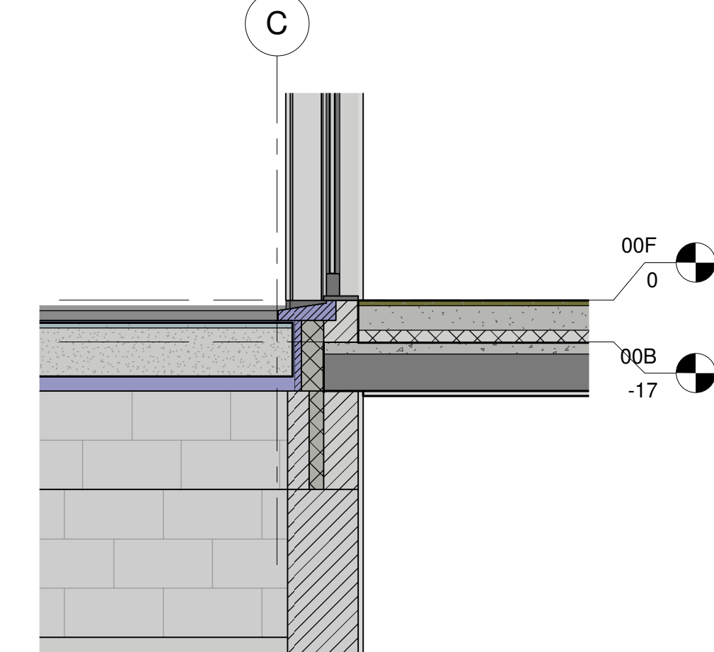
9 Coupe de détail 07 1 : 20
