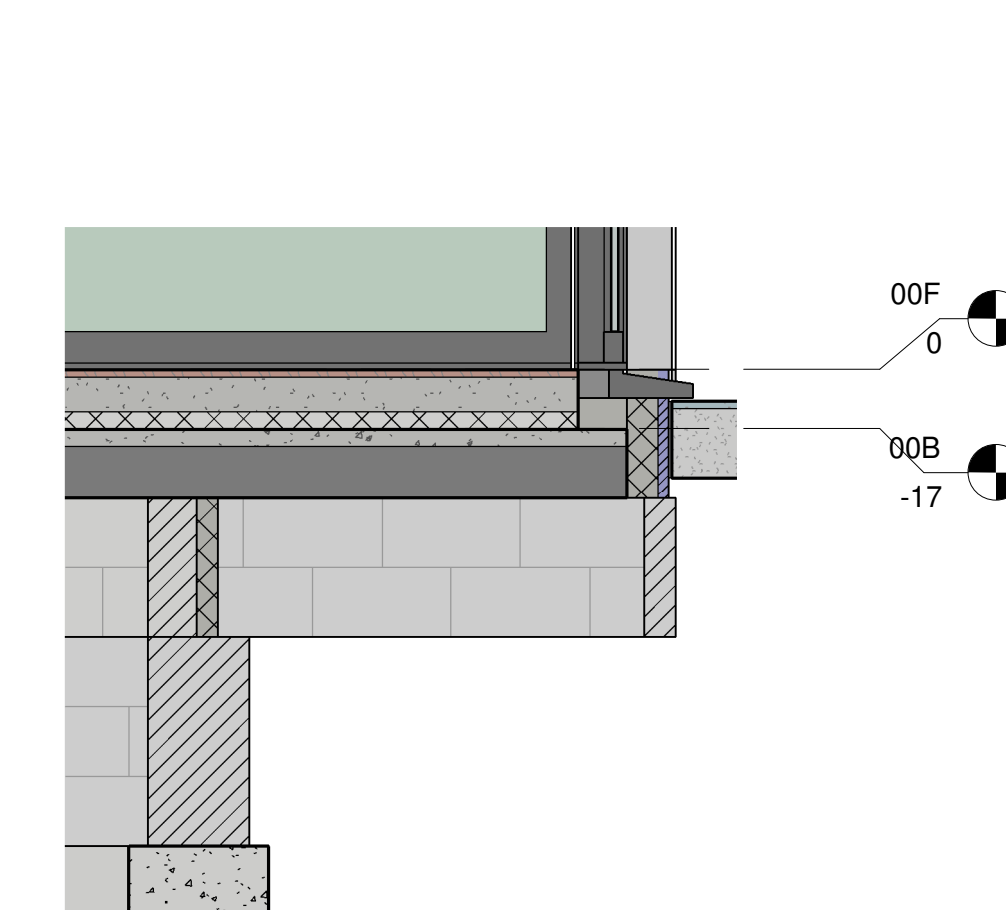
8 Coupe de détail 06 1 : 20
