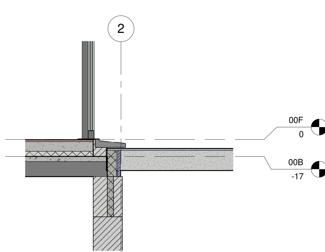
7 Coupe de détail 05 1 : 20
