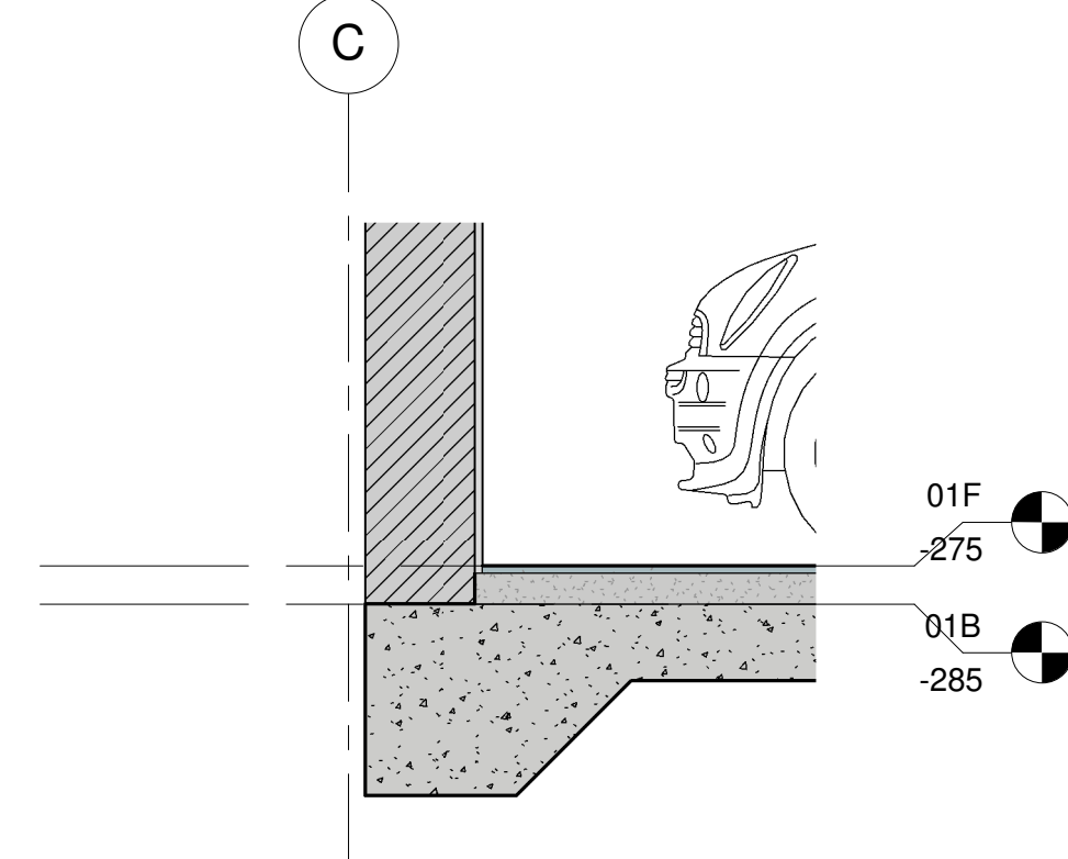
5 Coupe de détail 03 1 : 20
